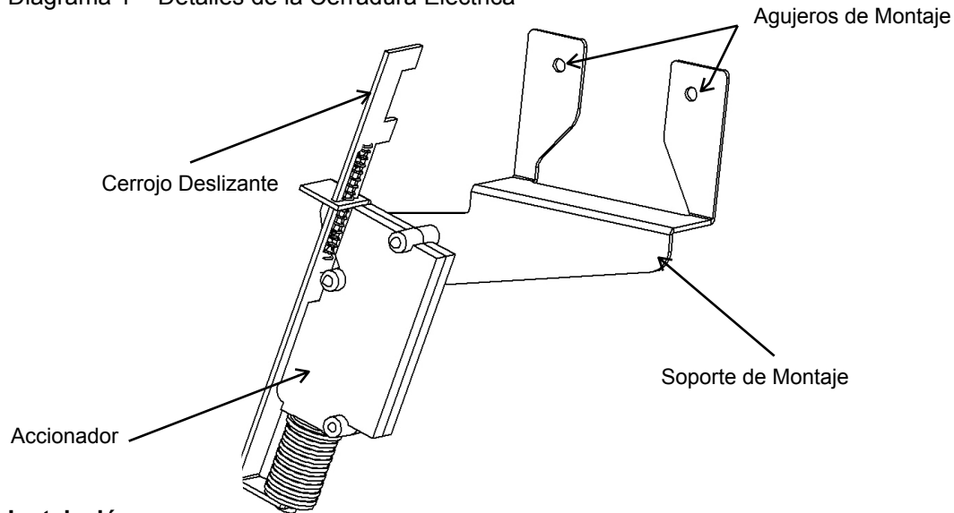
Diagrama 1 – Detalles de la Cerradura Eléctrica
